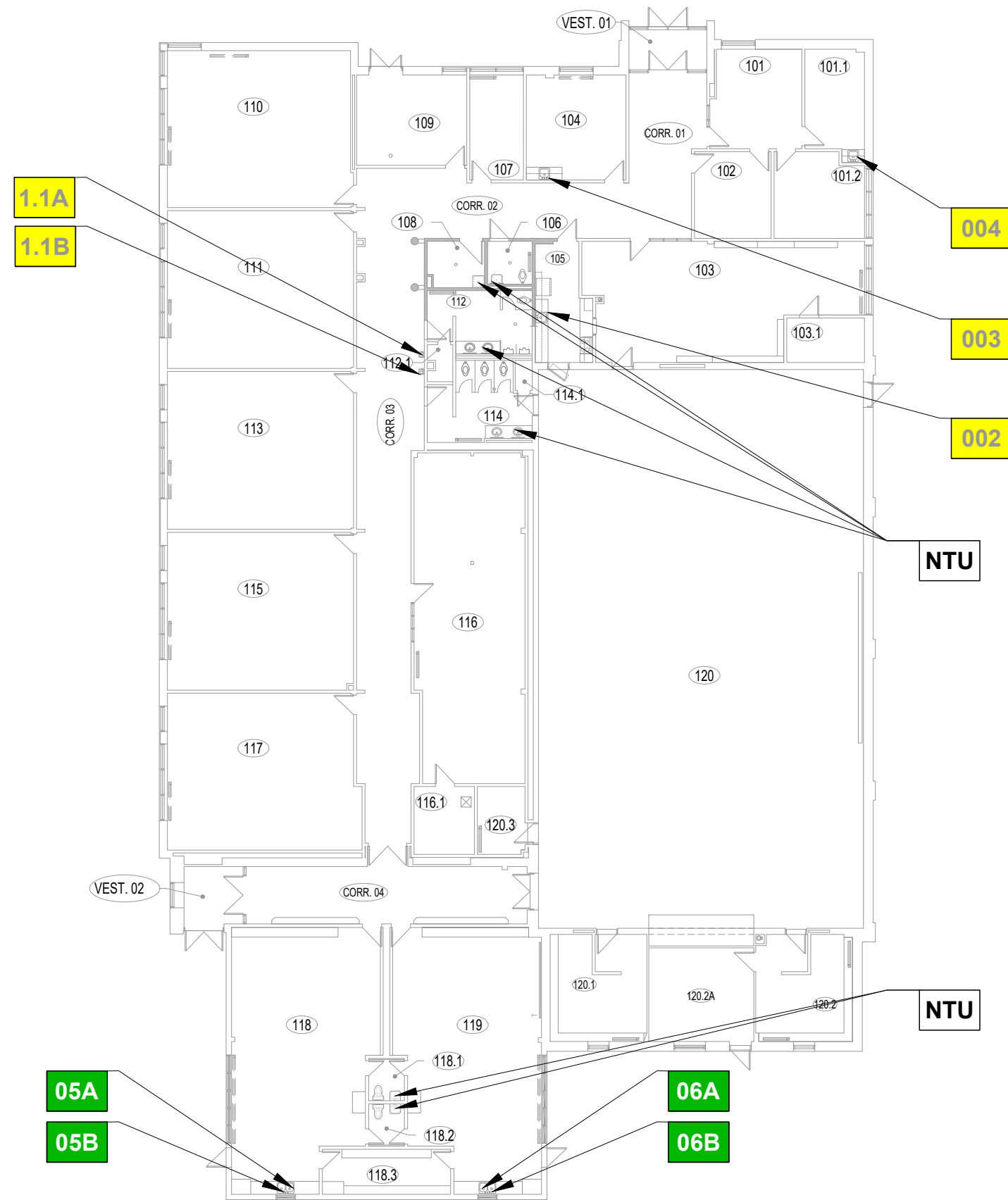
1 PLAN REZ-DE-CHAUSSÉE EAU-1 1:250
